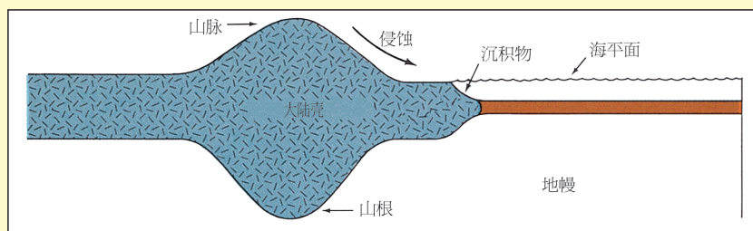
图 9： 另一张插图显示这些深根怎样使所在的山状似木桩。(Earth Science《地球科学》，作者塔巴克 (Tarbuck) 与陆得基 (Lutgens)，第 158 页。)
