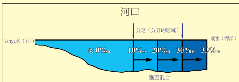
图 14: 显示河口中盐份 (千分之几 %) 纵截面。我们可从中看到淡水与咸水之间的分割 (分区区)。(《Introductory Oceanography 海洋学简介》, 作者塞门 (Thurman), 第 301 页, 稍有修改。)
