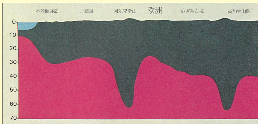
图 8： 截面示意图。 状似木桩的山有植入土地深根。(Anatomy of the Earth《地球结构》，作者西里士 (Cailleux)，第 220 页。)
