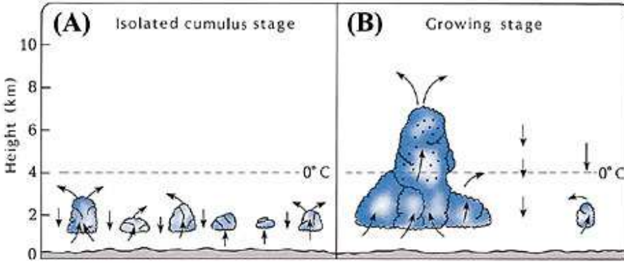
Şekil 19: (A) İzole edilmiş bulut parçaları (kümüls bulutları), (B) Küçük bulutlar birleştiği zaman, büyük bulutun içindeki üstteki akışlar artar, böylece bulut üst üste istiflenir. Yağmur, su damlaları ile gösterilmiştir 29 . (Atmosfer, Antles ve arkadaşları, Sayfa 268-269)
