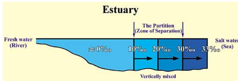
Figuur 14: Overlangse doorsnede van een estuarium laat de zoutdichtheid (gedeeltes zijn in promille (‰) weergegeven) zien. We kunnen hier de vakjes (scheidingszone) tussen het zoete en het zoute water zien. ( Introductory Oceanography , Thurman, p.301, enigszins vergroot).
