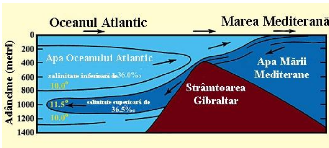
Figura 13. Apa Mării Mediterane intră în oceanul Atlantic prin strâmtoarea Gibraltar, păstrându-și propria temperatură, salinitate și densitate mică, datorită barierei care separă cele două ape. Temperaturile sunt exprimate în grade Celsius. ( Geologia marină , Kuenen, p. 43)
