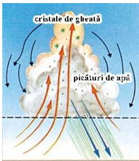
Figura 20. Nor cumulonimbus . După ce norul crește, ploaia iese din el. ( Timpul și clima , Bodin, p.123)
