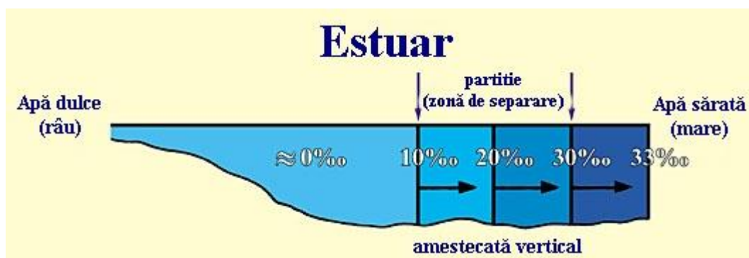
Figura 14. Secțiune longitudinală care arată salinitatea în estuar. Putem observa zona de separare dintre apa dulce și cea sărată. ( Introducere în oceanografie , Thurman, p. 301)
