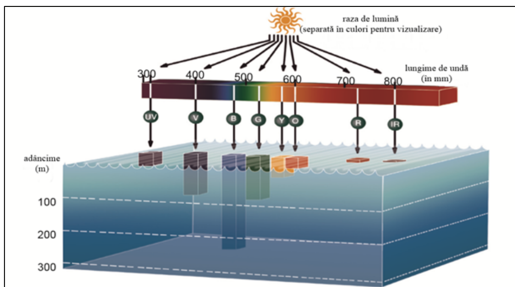
Figura 15. Între 3 și 30% din lumina solară este reflectată de suprafața mării. Astfel, aproape toate cele șapte culori ale spectrului solar sunt absorbite una după alta în primii 200 de metri, în afară de lumina albastră. ( Oceanele , Elder și Pernetta, p. 27).
