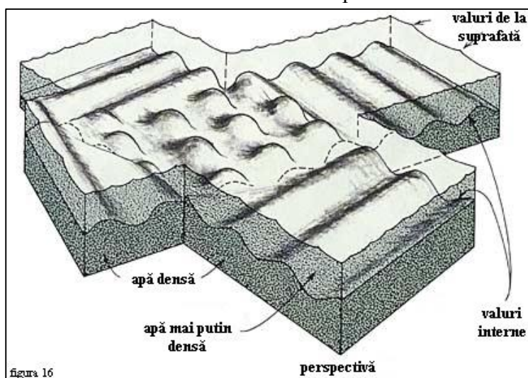
Figura 16. Valuri interne în zona limitofă dintre două straturi de apă cu densități diferite. Unul este dens (cel inferior) și celălalt este mai
