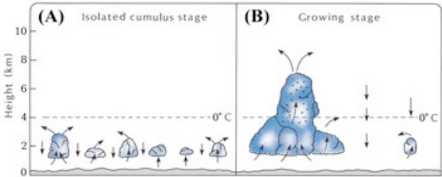
Εικόνα 19: (A) Απομονωμένα μικρά τμήματα σύννεφων (σωρειτών). (B) Όταν τα μικρά σύννεφα ενώνονται, τα ανοδικά ρεύματα μέσα στα μεγαλύτερα σύννεφα αυξάνονται, κι έτσι το σύννεφο συσσωρεύεται. Οι σταγόνες νερού απεικονίζονται με •. [ The Atmosphere (Η Ατμόσφαιρα), Anthes και άλλοι, σελ. 269.]
