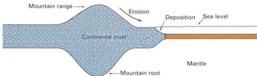
Εικόνα 9: Άλλη μία απεικόνιση δείχνει πως τα βουνά έχουν το σχήμα πασσάλου, εξαιτίας των βαθιών ριζών τους. [ Earth Science (Επιστήμες της Γης), Tarbuck και Lutgens, σελ. 158].
