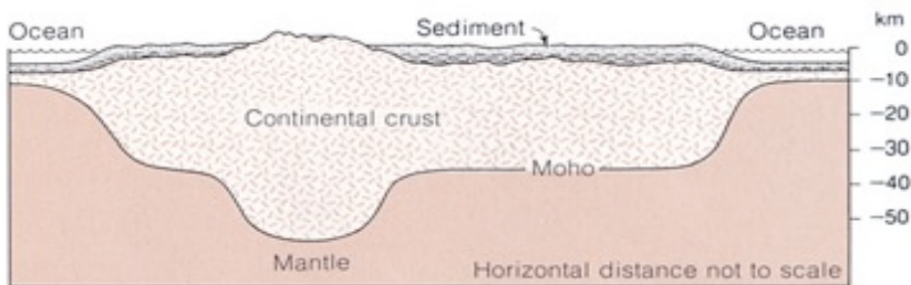
Εικόνα 7: Τα βουνά έχουν βαθιές ρίζες κάτω από την επιφάνεια του εδάφους [ Earth (Γη), Press και Siever, σελ. 413.]
