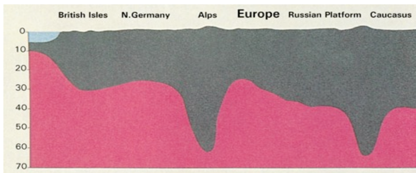
Εικόνα 8: Σχηματική τομή. Τα βουνά, σαν πάσσαλοι, έχουν βαθιές ρίζες ενσωματωμένες στο έδαφος [ Anatomy of the Earth (Ανατομίας της Γης), Cailleux, σελ. 220].
